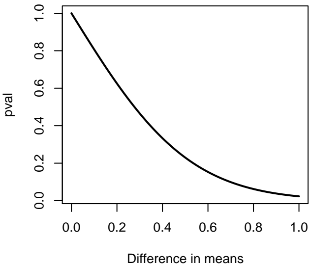
P-value
